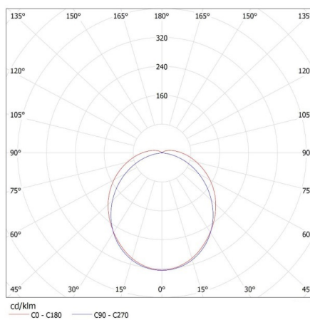
KANLUX S.A. (kat 22607) MAH LED HI 38W-NW RYF / LDC (Polar)
