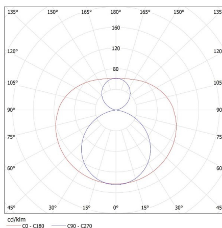
MILED0 (kat 31193) T8 N LED 9W-CW / LDC (Polar)
